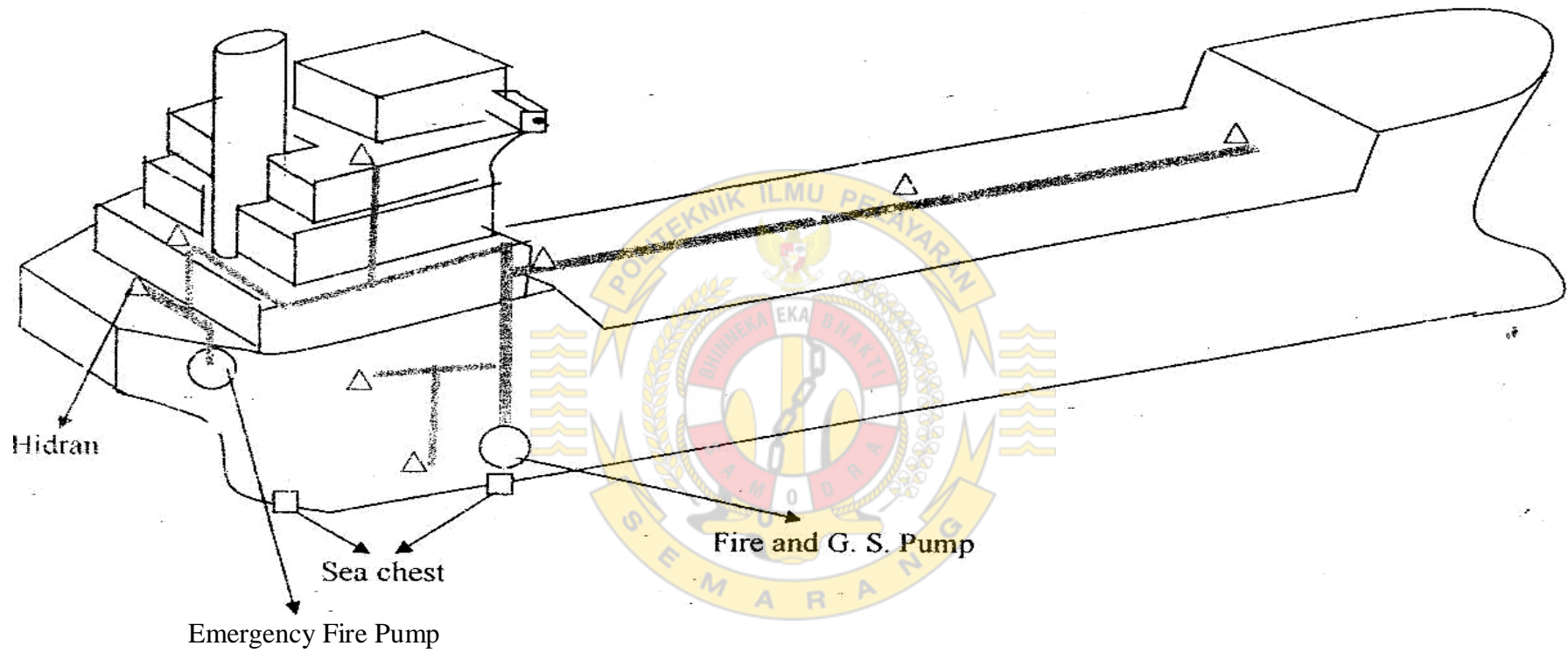
Gambar 8. Penataan pipa Pemadam Kebakaran di Kapal MT. Sinar Jogya
