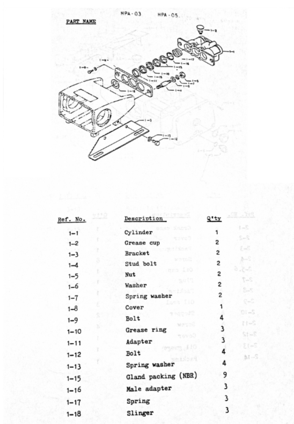
GAMBAR: BAGIAN LIQUID END
