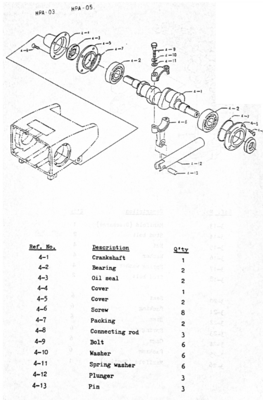
GAMBAR: BAGIAN POWER END
