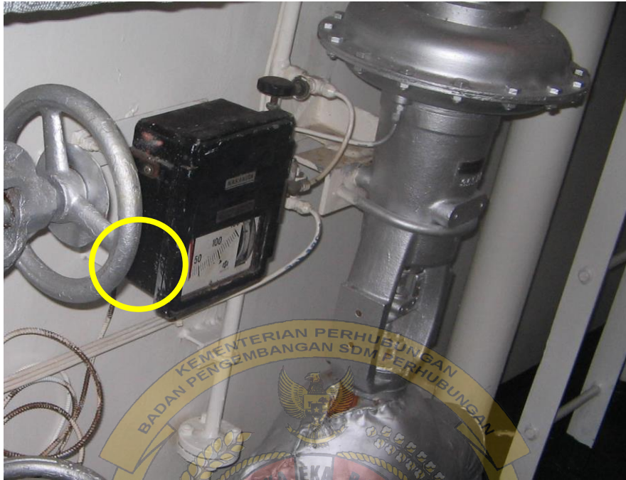
Gambar 1. Penunjuk temperatur air yang telah dipanaskan oleh tank cleaning heater menunjukkan tidak lebih dari 50 0 C.
