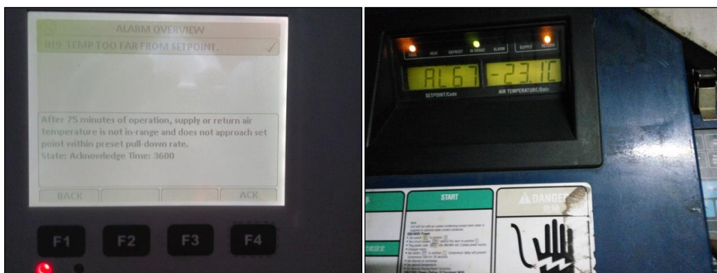
Gambar 9 contoh alarm yang muncul pada reefer container ketika pengecekan rutin
