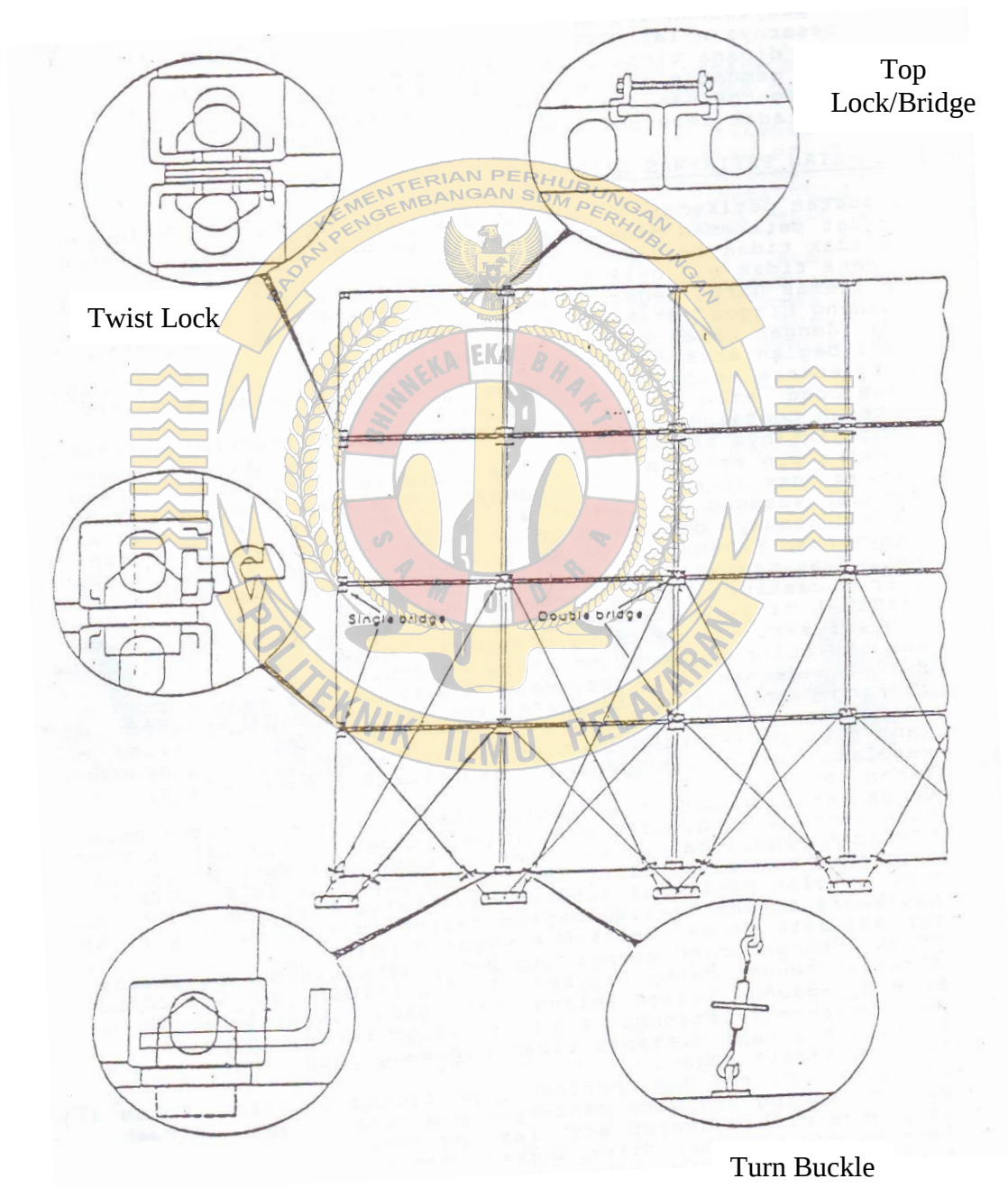
Gambar I. Sistem Pelashingan Container di Deck
