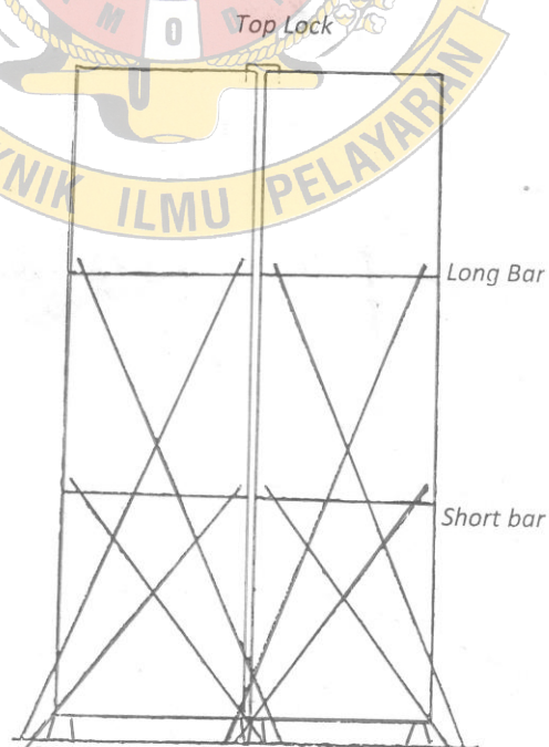
Gambar 4. Pelashingan Tiga Tier
