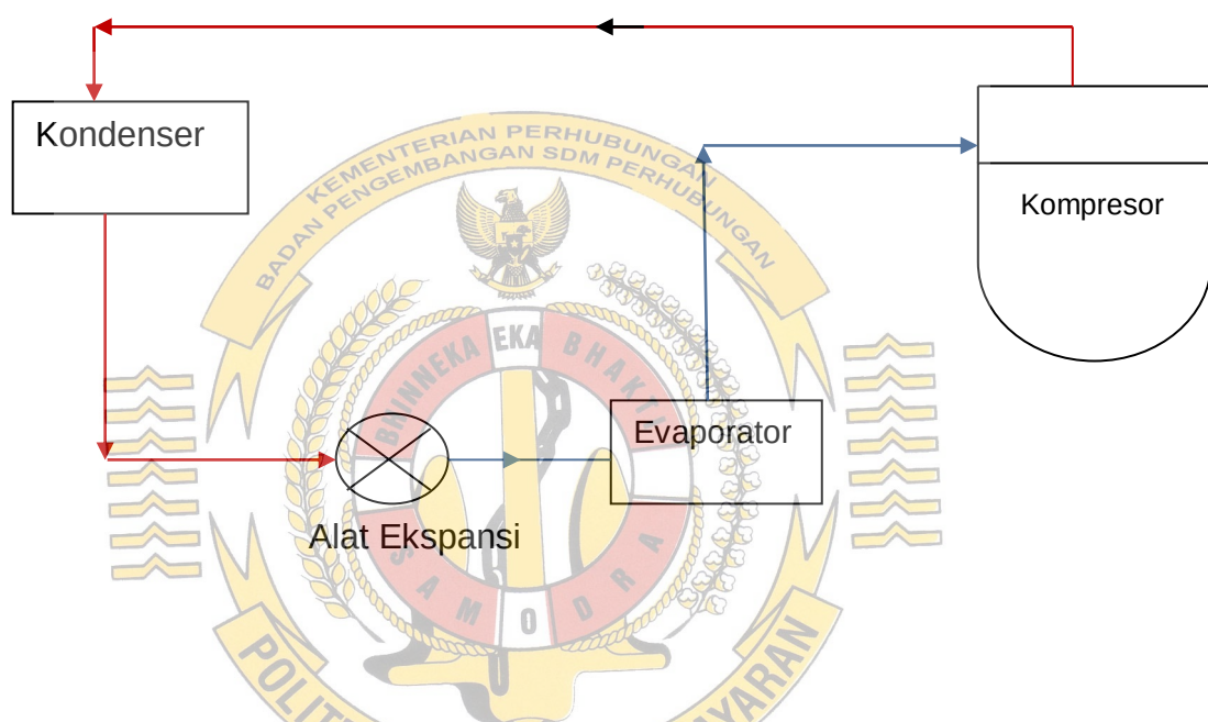
Gambar. Perpipaan pada sistem refrigerasi
