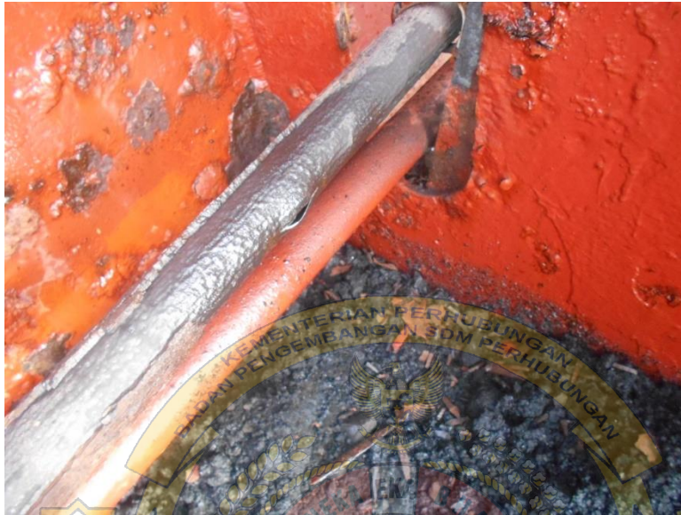
Gambar 1 Pipa yang hidrolik ke jack yang pecah
