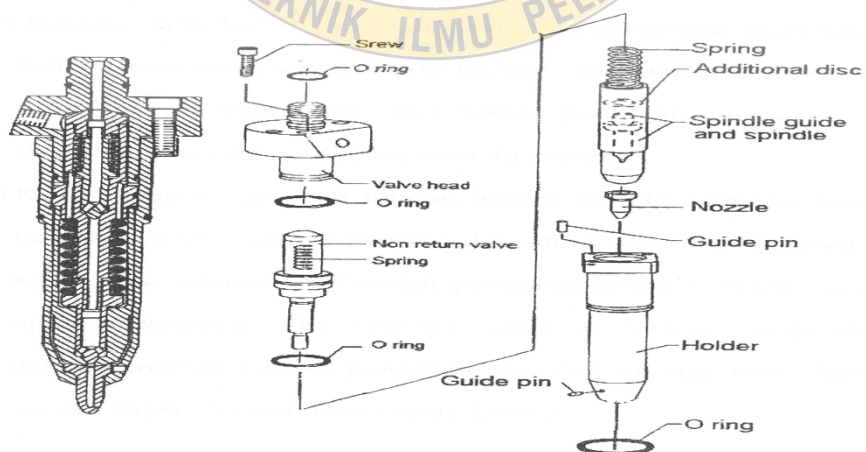
Gambar 4.6 Komponen Injector
