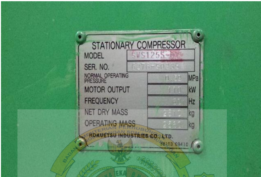
Gambar plat kompresor udara
