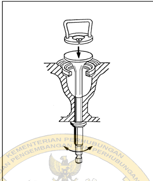
Gambar 9 Cara pembaharuan permukaan katup secara manual
