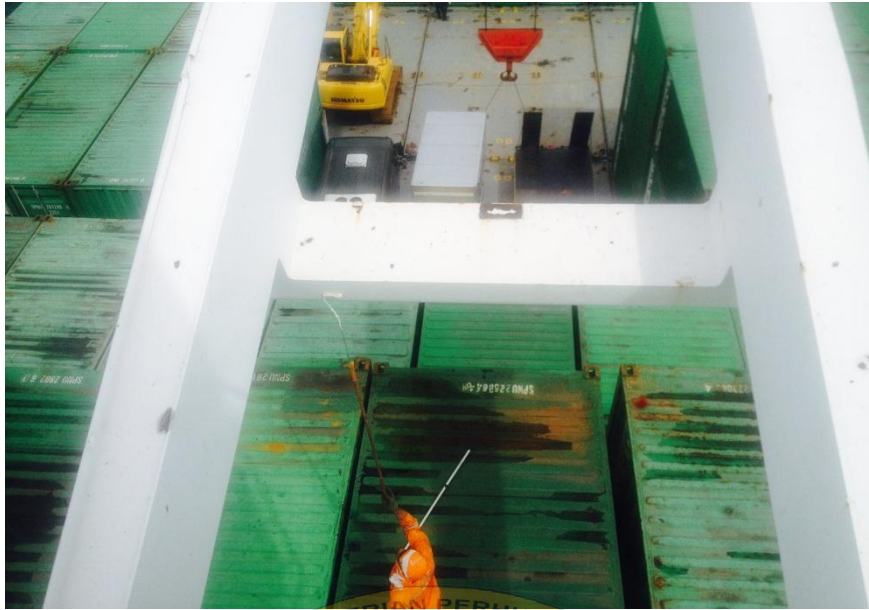
Gambar 4.3 Pengecatan batang pemuat crane
