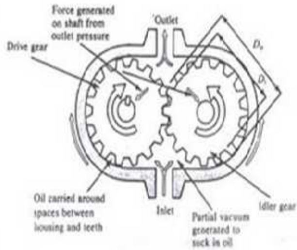
Gambar: Pompa roda gigi Di KM. Gunung Dempo
