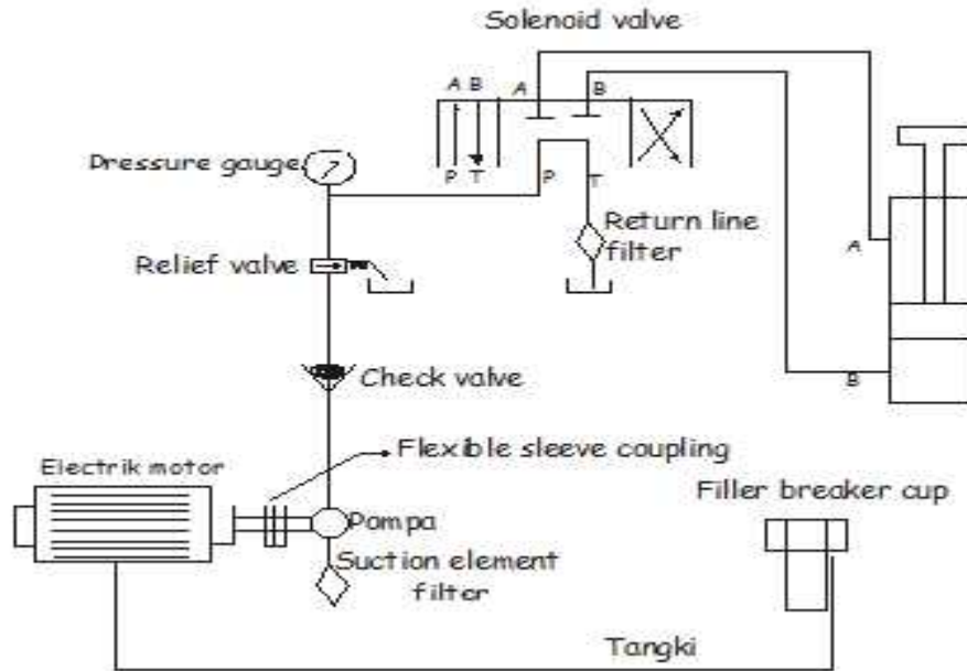
Gambar: Hydraulic Sytem Di KM.Gunung Dempo
