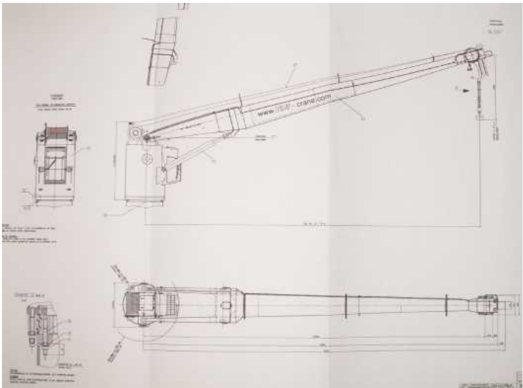
Gambar Crane Hydraulic di KM. Gunung Dempo
