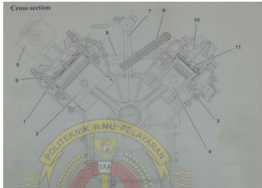
Gambar 2.2 : Kompresor udara dua tingkat tekan
