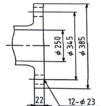
DIS. FLANGE JIS 5K-250A
